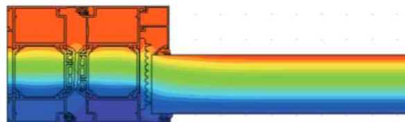
Rozkład temperatur
