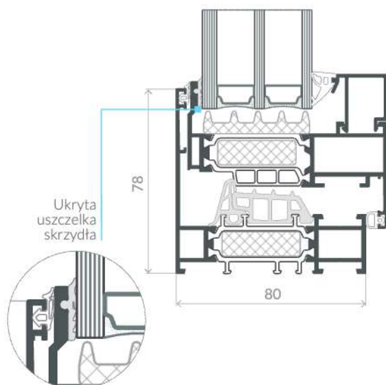
Przekrój przez okno otwierane z ukrytym skrzydłem
