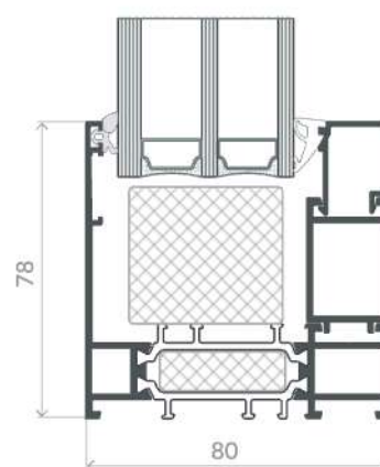
Przekrój przez kwaterę stałą okna z ukrytym skrzydłem
